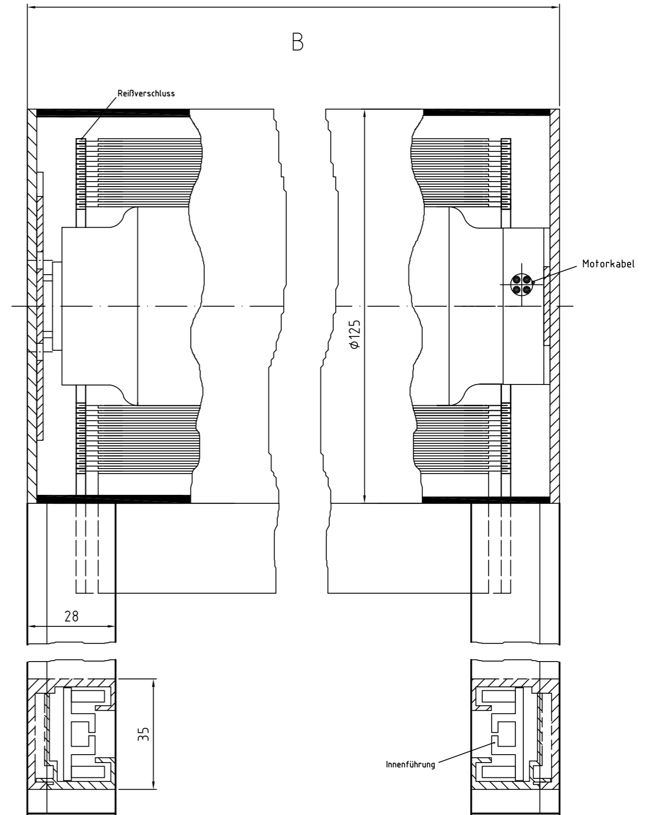
Zeichnung SM-ZIP-MR – Längsschnitt Systemskizze | ohne Maßstab | sämtliche Angaben in mm
