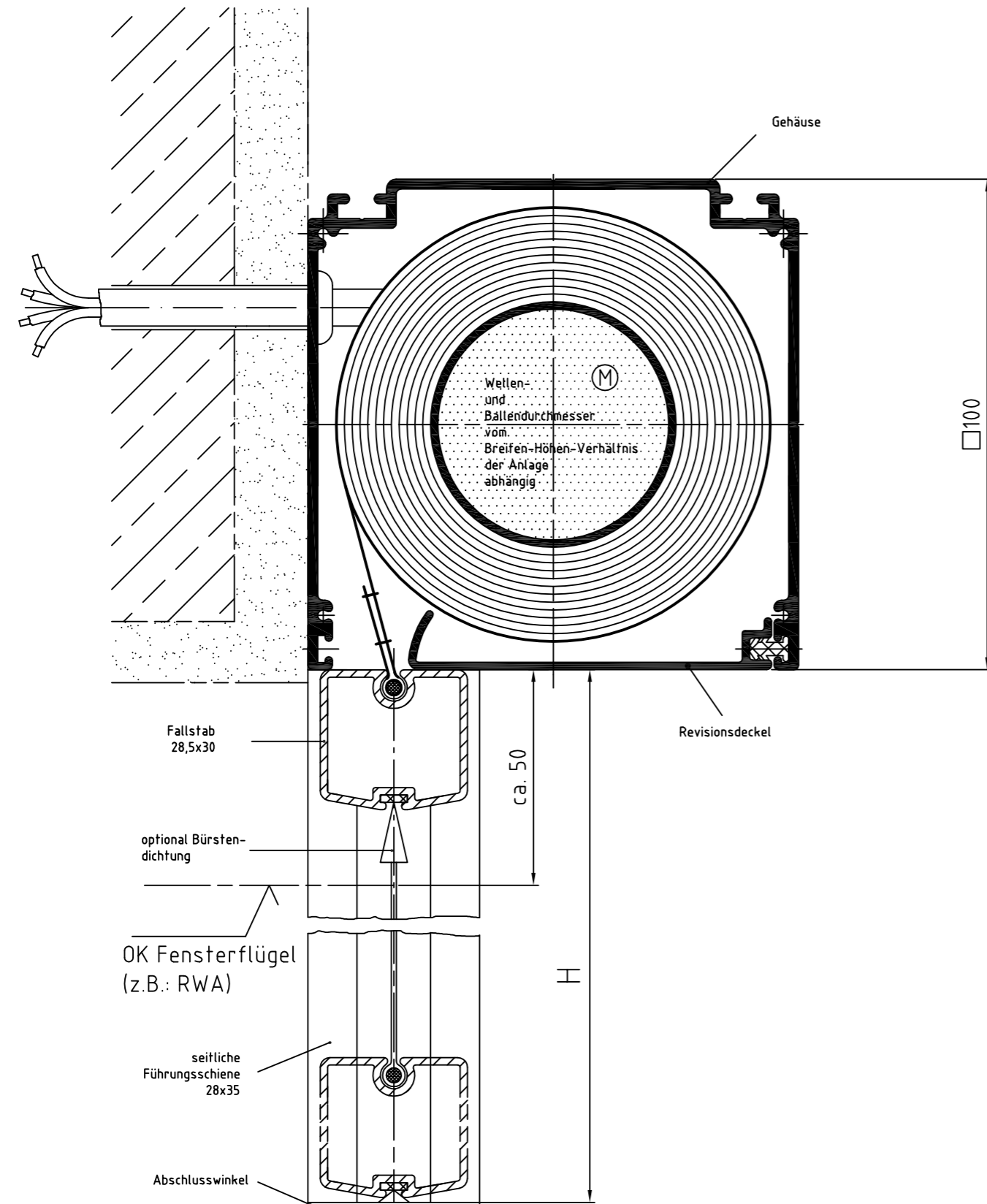
Zeichnung SM-ZIP-MQ 100 – Querschnitt Systemskizze | ohne Maßstab | sämtliche Angaben in mm
