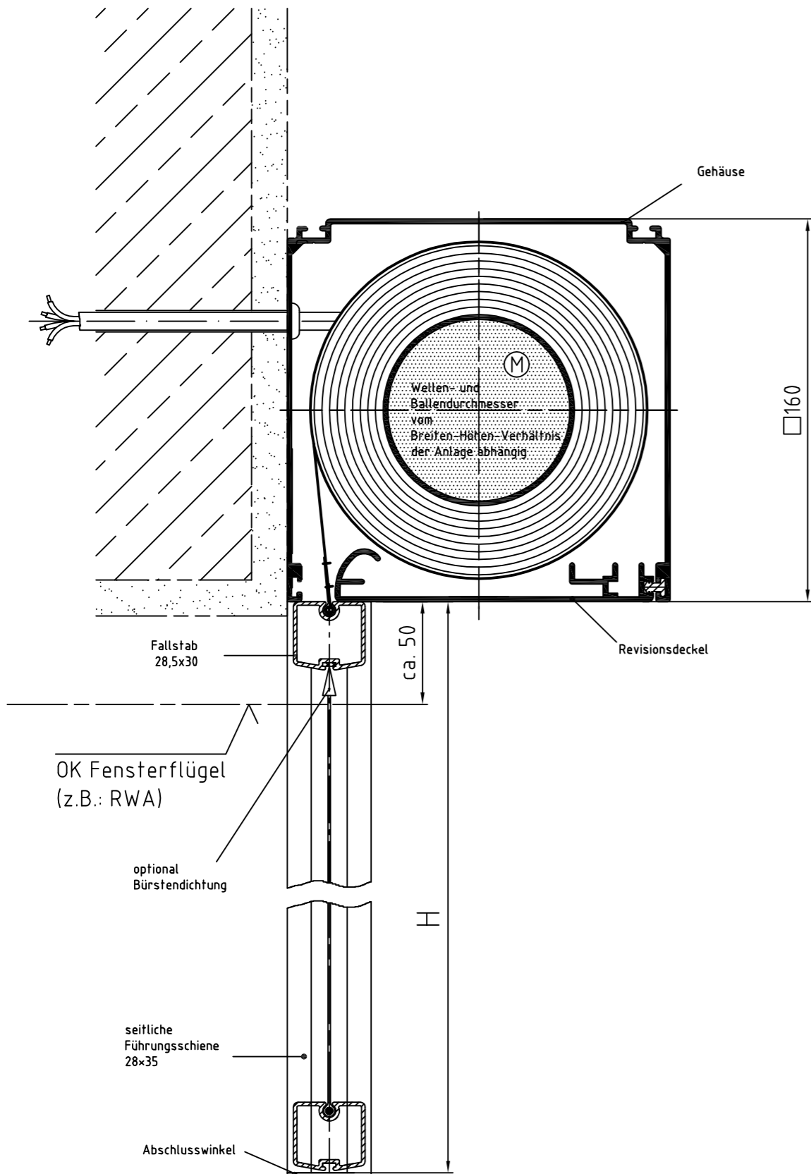
Zeichnung SM-ZIP-MQ 160 – Querschnitt Systemskizze | ohne Maßstab | sämtliche Angaben in mm
