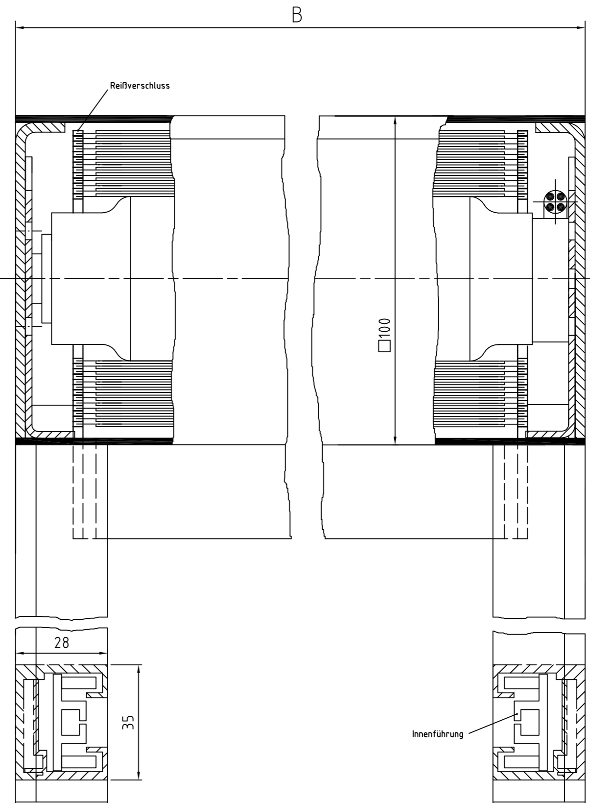
Zeichnung SM-ZIP-MQ 100 – Längsschnitt Systemskizze | ohne Maßstab | sämtliche Angaben in mm
