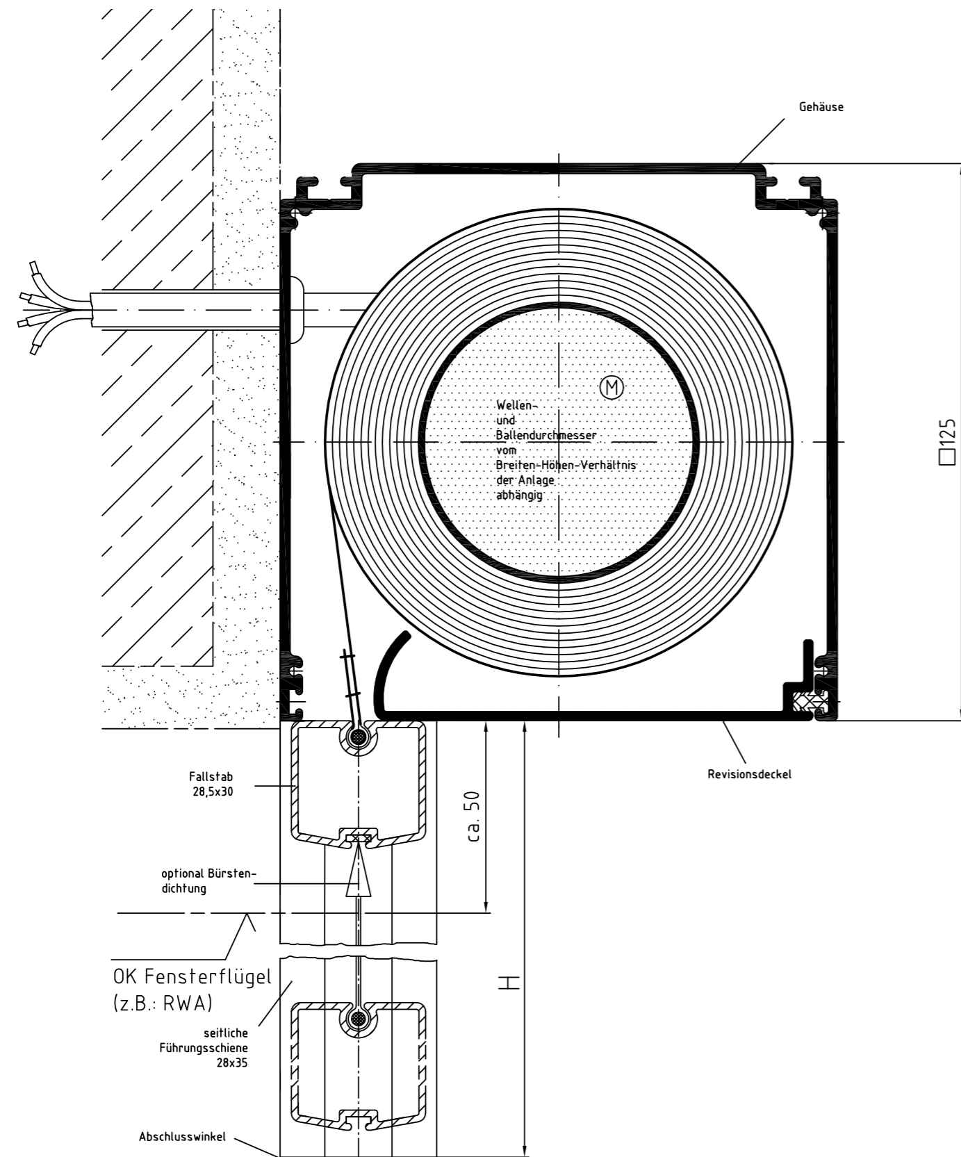
Zeichnung SM-ZIP-MQ 125 – Querschnitt Systemskizze | ohne Maßstab | sämtliche Angaben in mm
