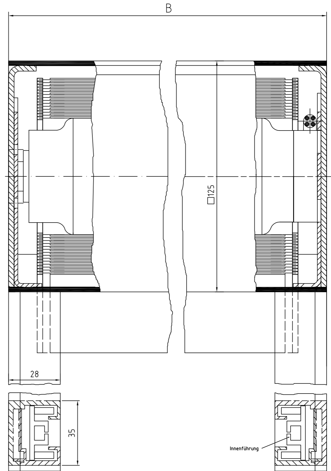
Zeichnung SM-ZIP-MQ 125 – Längsschnitt Systemskizze | ohne Maßstab | sämtliche Angaben in mm
