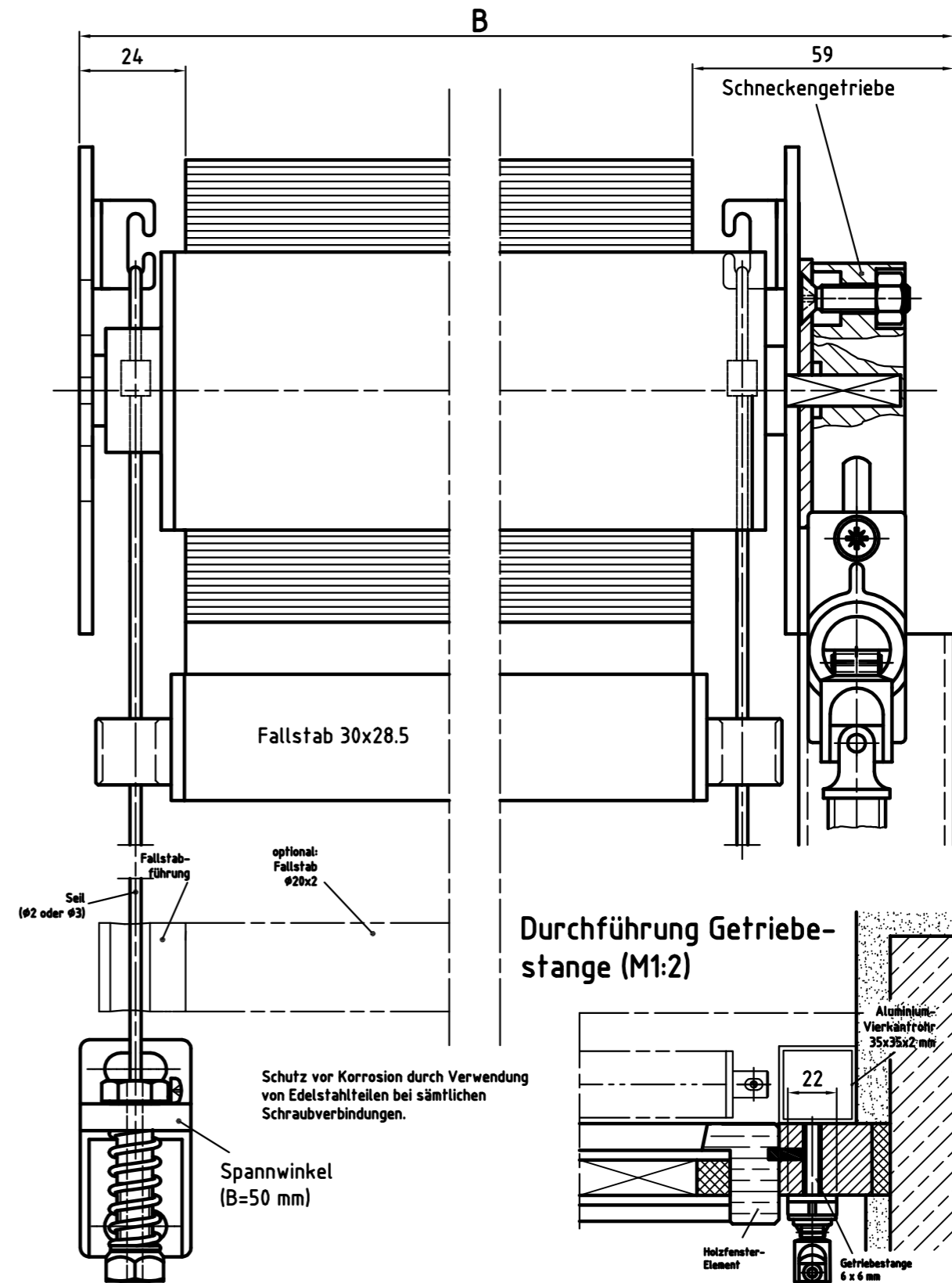
Zeichnung SM-GO – Längsschnitt Systemskizze | ohne Maßstab | sämtliche Angaben in mm
