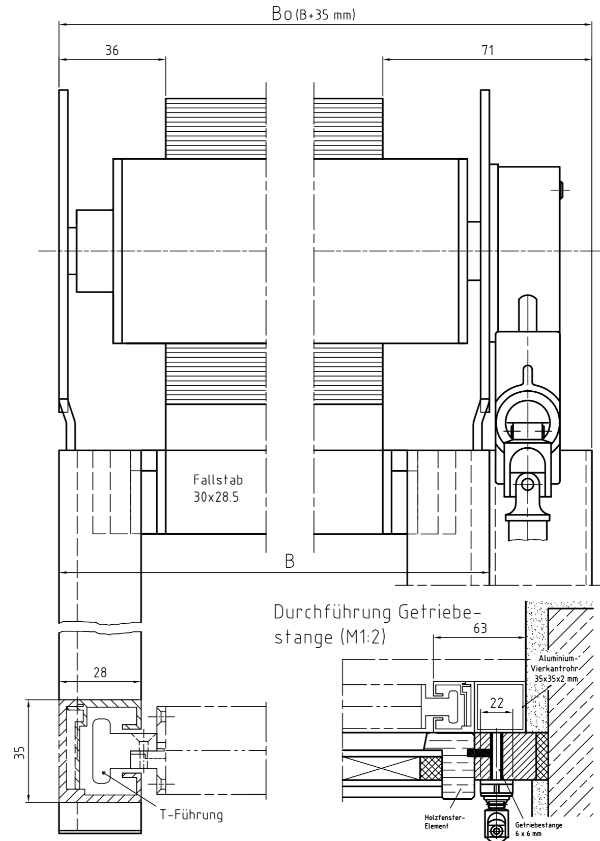
Zeichnung SM-GO – Längsschnitt Systemskizze | ohne Maßstab | sämtliche Angaben in mm
