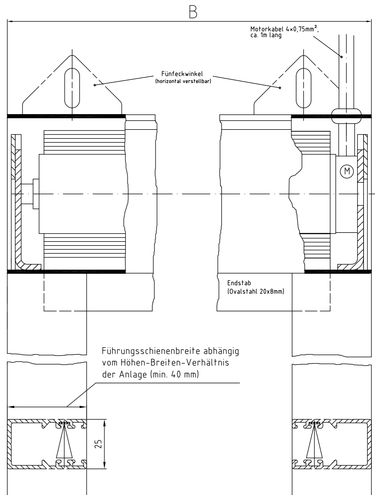
Zeichnung L-MQ 80 – Längsschnitt Systemskizze | ohne Maßstab | sämtliche Angaben in mm
