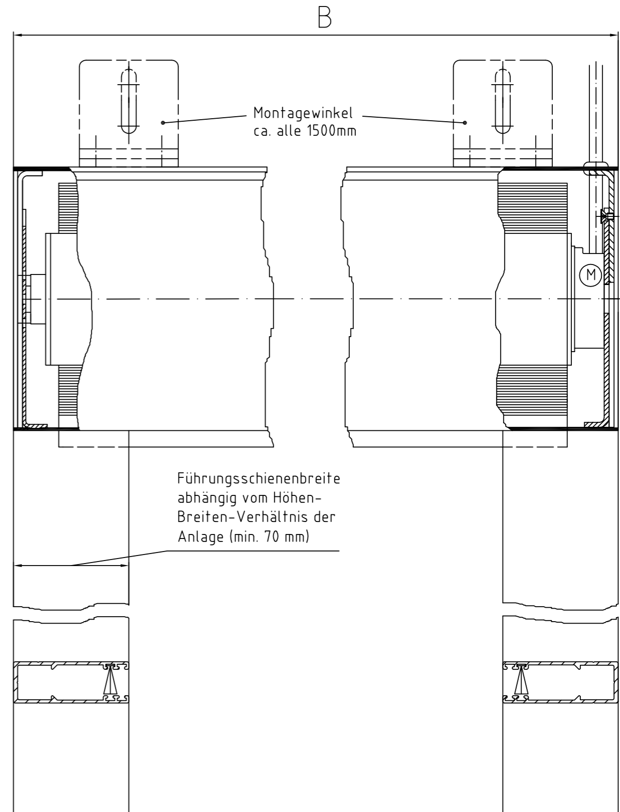
Zeichnung L-MQ 160 – Längsschnitt Systemskizze | ohne Maßstab | sämtliche Angaben in mm
