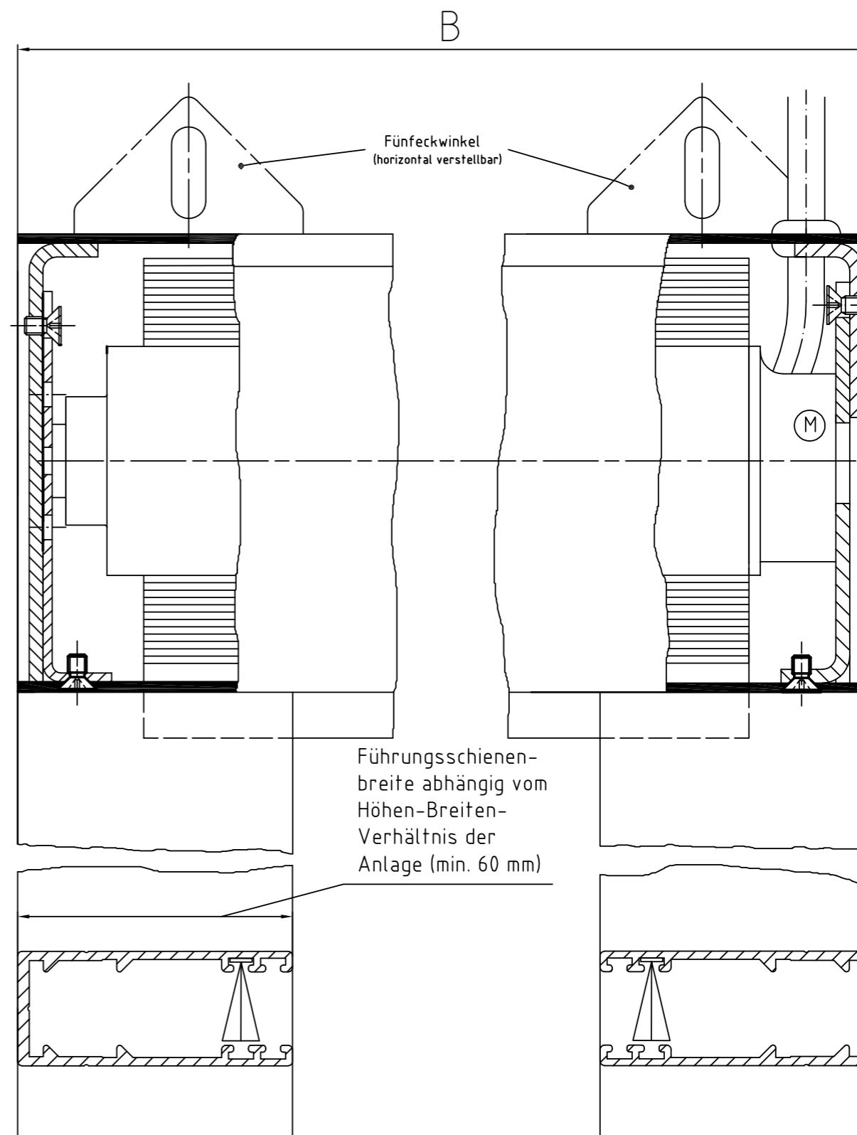
Zeichnung L-MQ 100 – Längsschnitt Systemskizze | ohne Maßstab | sämtliche Angaben in mm
