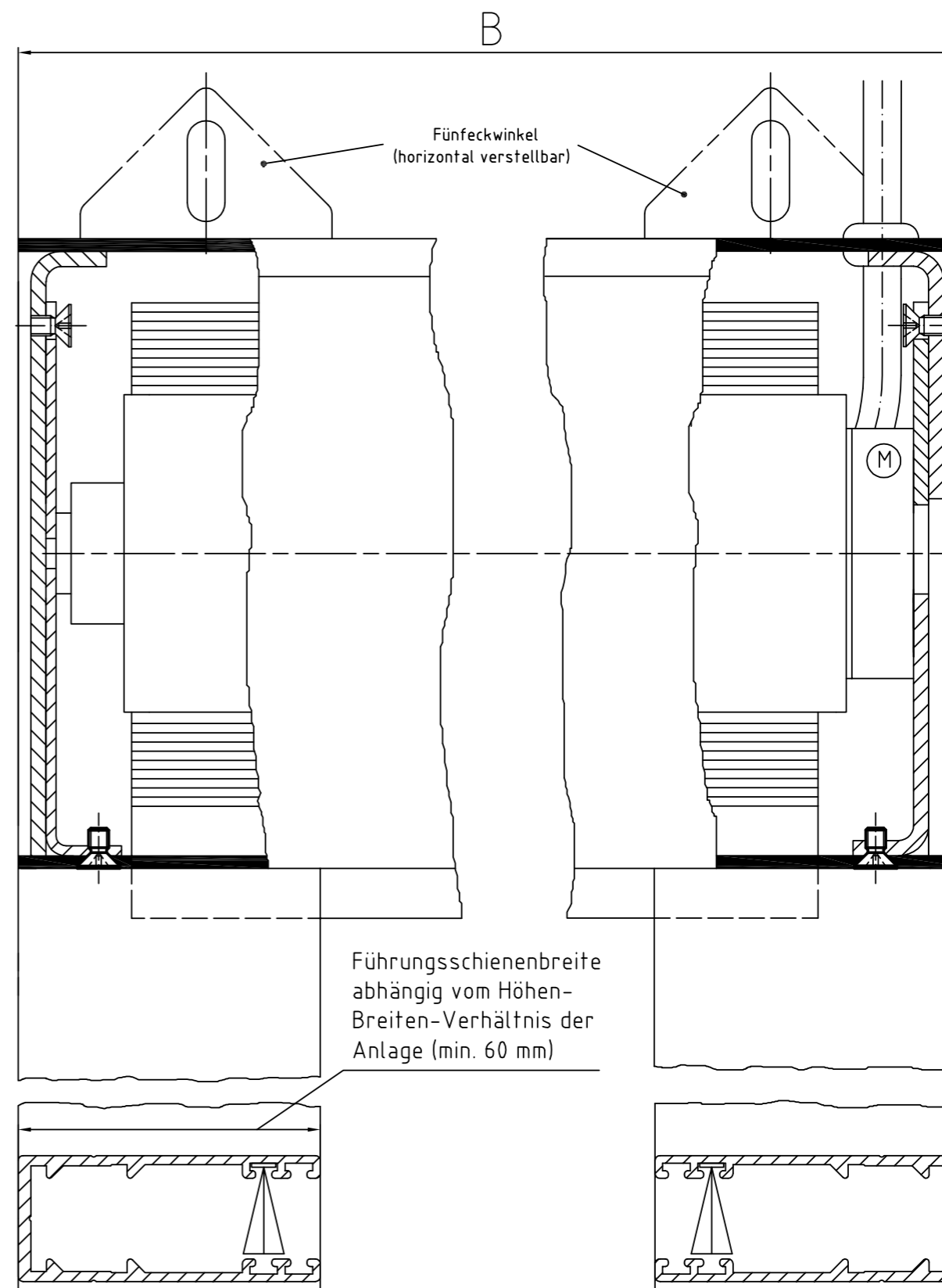
Zeichnung L-MQ 125 – Längsschnitt Systemskizze | ohne Maßstab | sämtliche Angaben in mm
