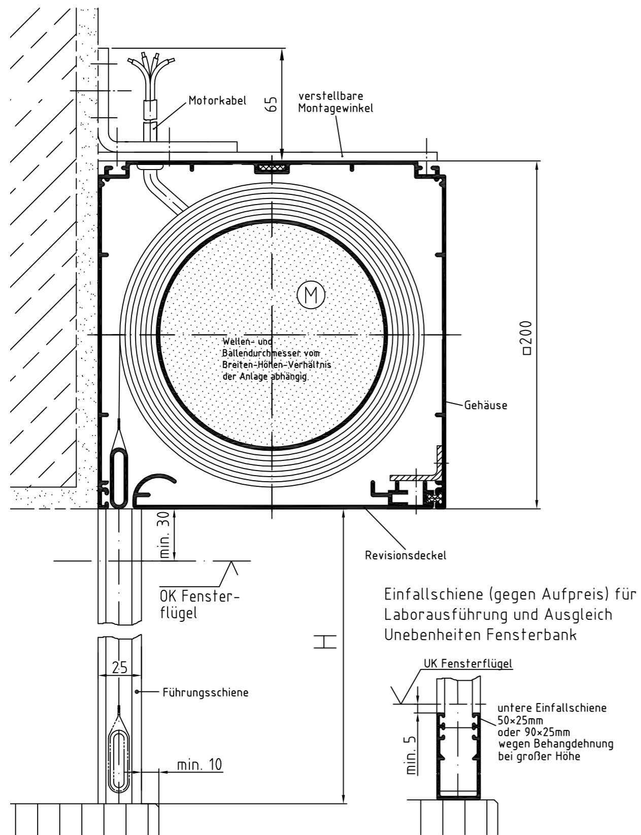
Zeichnung L-MQ 200 – Querschnitt Systemskizze | ohne Maßstab | sämtliche Angaben in mm
