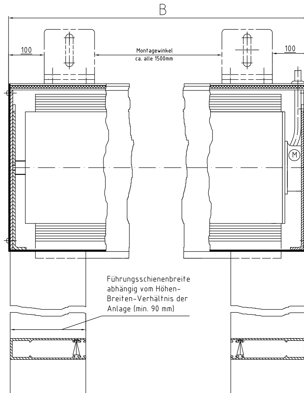
Zeichnung L-MQ 200 – Längsschnitt Systemskizze | ohne Maßstab | sämtliche Angaben in mm
