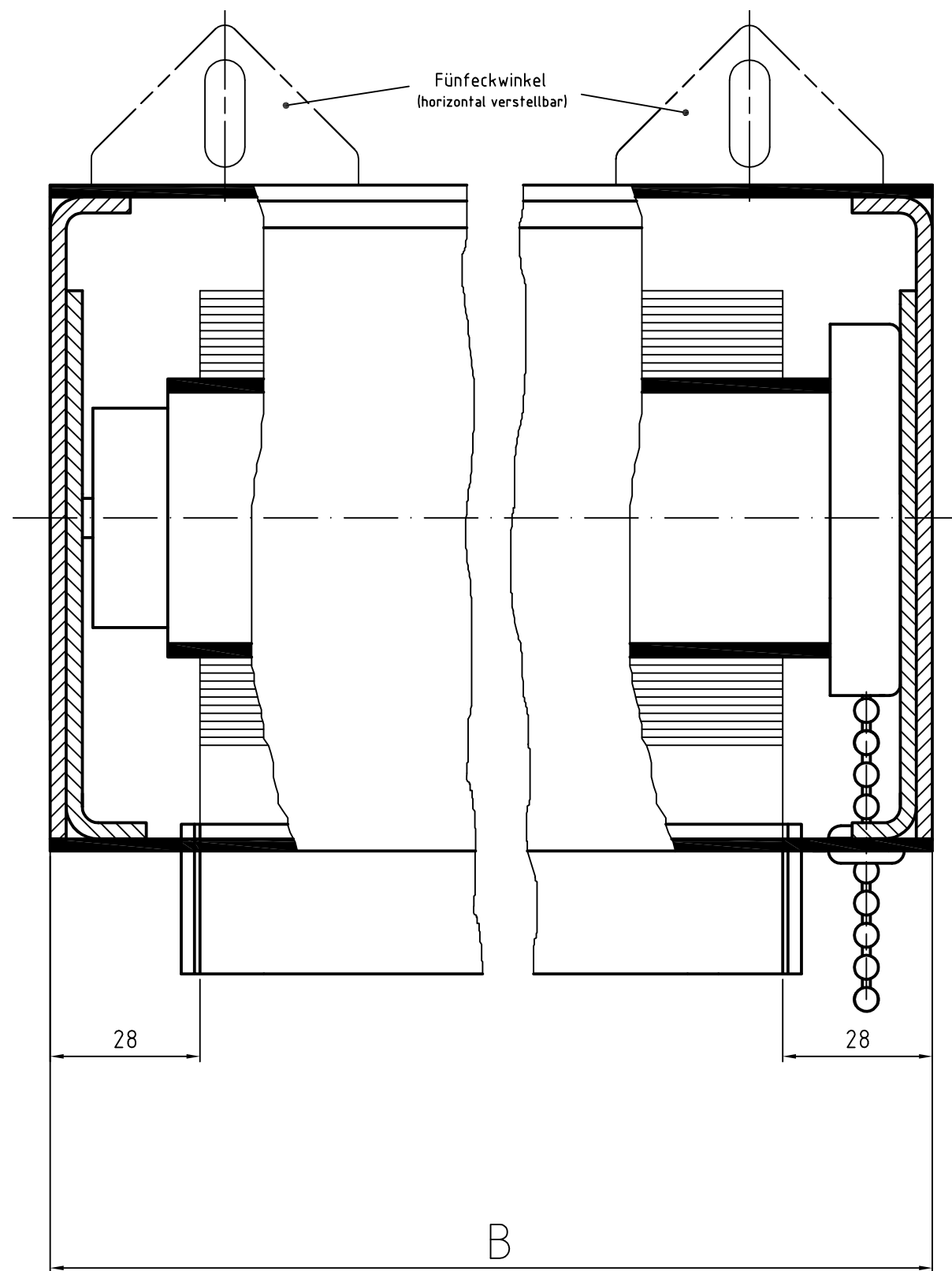
Zeichnung L-KQ 125 – Längsschnitt Systemskizze | ohne Maßstab | sämtliche Angaben in mm
