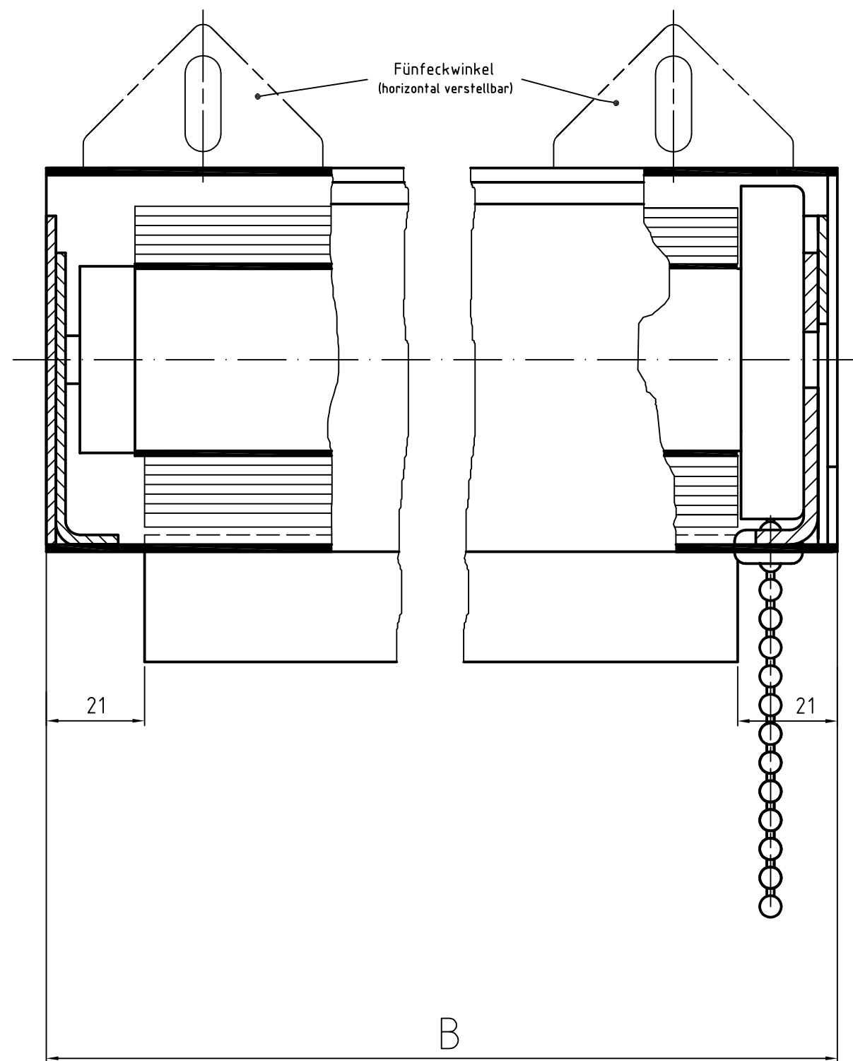
Zeichnung L-KQ 80 – Längsschnitt Systemskizze | ohne Maßstab | sämtliche Angaben in mm
