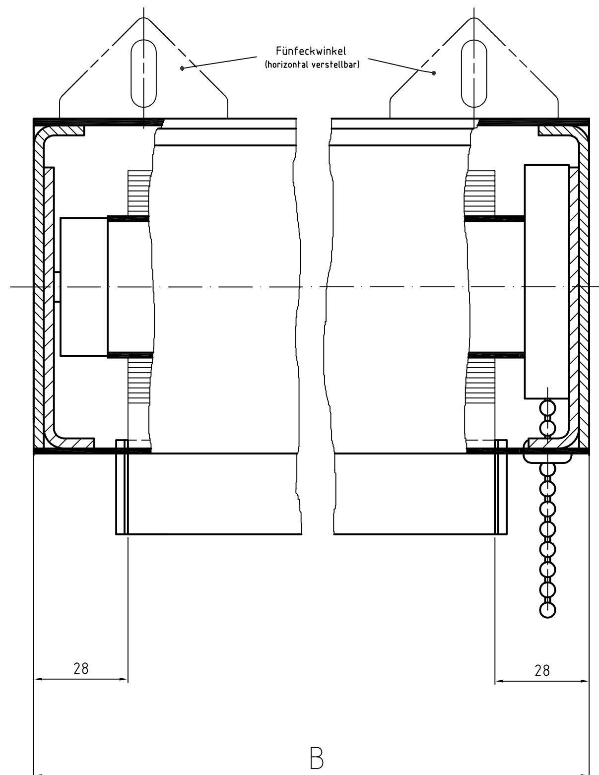
Zeichnung L-KQ 100 – Längsschnitt Systemskizze | ohne Maßstab | sämtliche Angaben in mm
