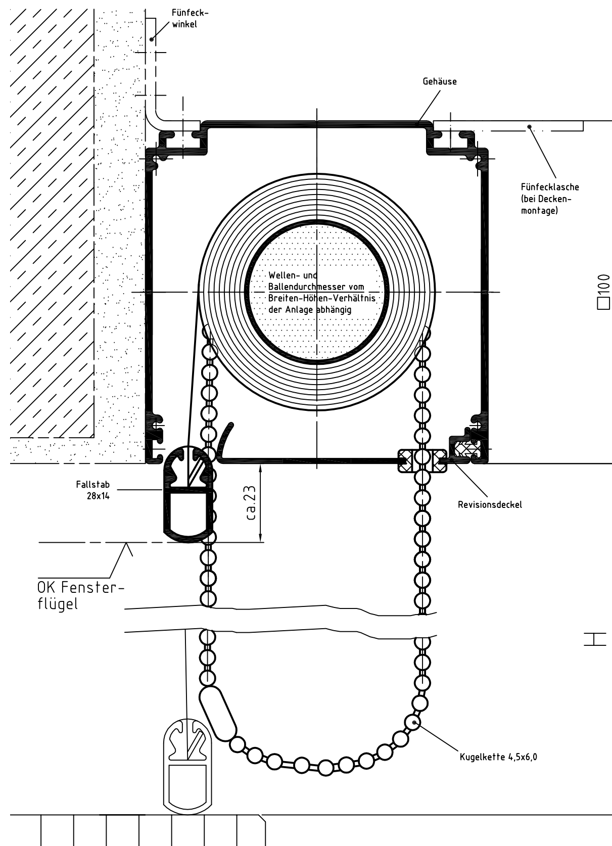
Zeichnung L-KQ 100 – Querschnitt Systemskizze | ohne Maßstab | sämtliche Angaben in mm
