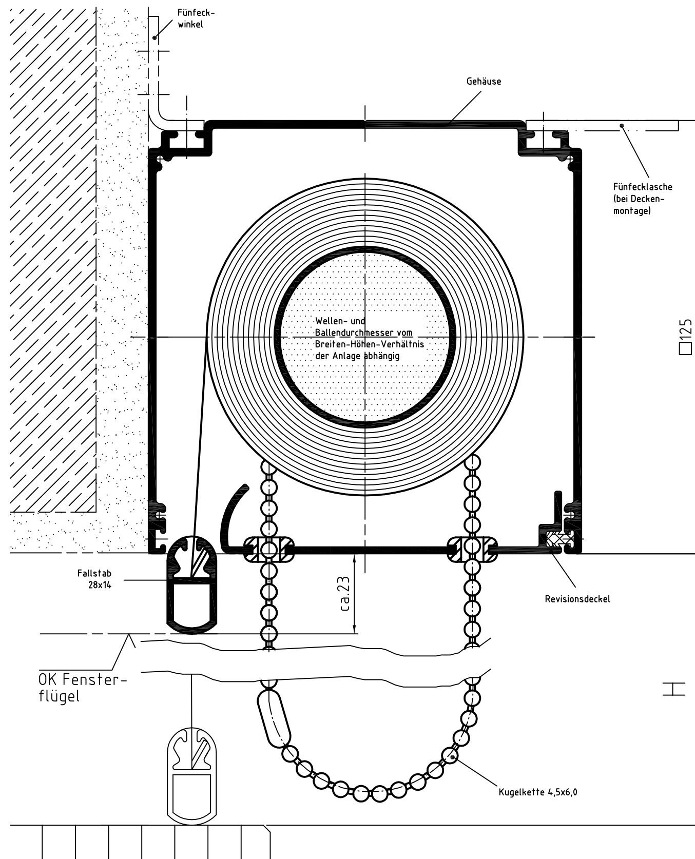
Zeichnung L-KQ 125 – Querschnitt Systemskizze | ohne Maßstab | sämtliche Angaben in mm
