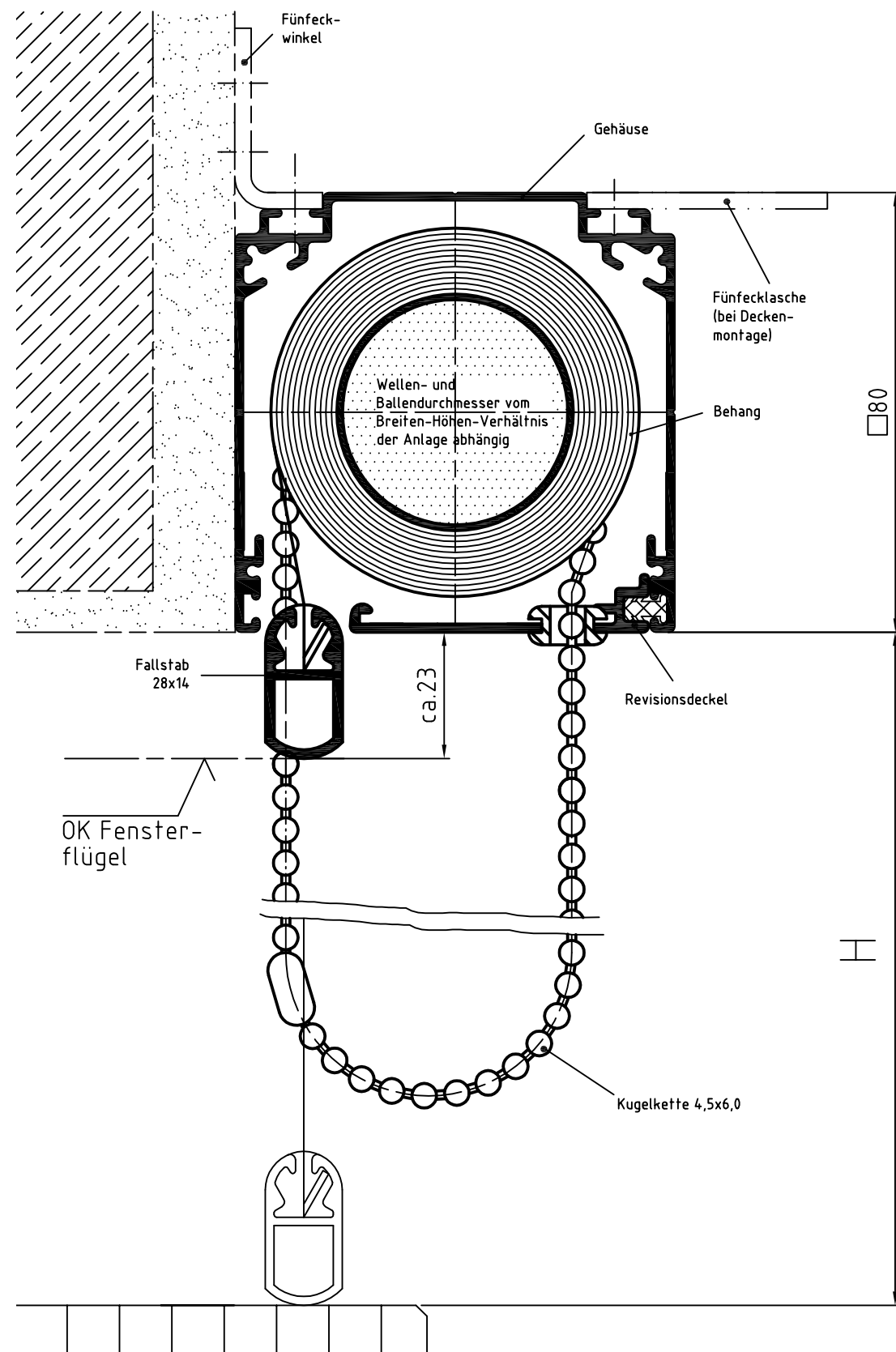
Zeichnung L-KQ 80 – Querschnitt Systemskizze | ohne Maßstab | sämtliche Angaben in mm
