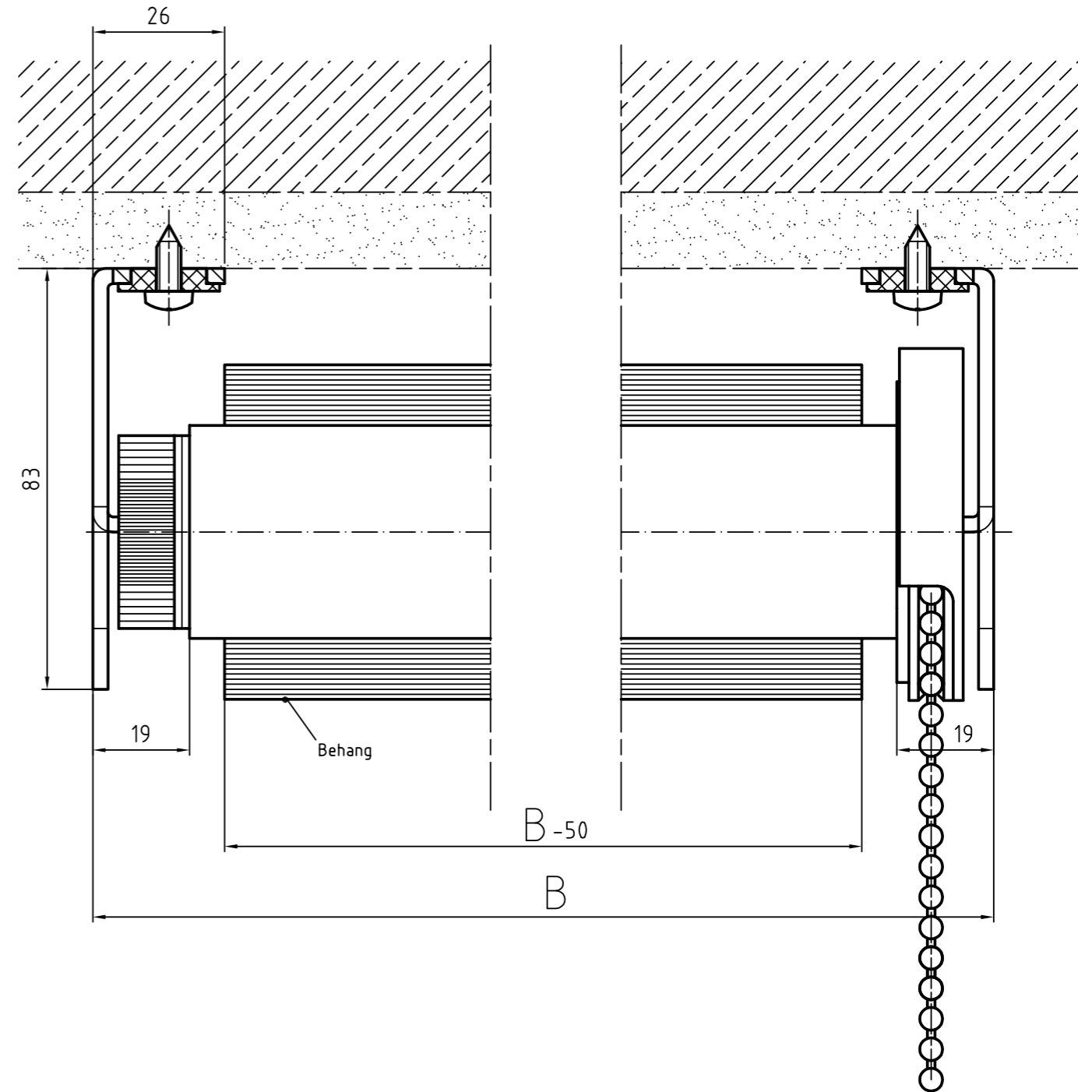
Zeichnung L-KO – Längsschnitt Systemskizze | ohne Maßstab | sämtliche Angaben in mm
