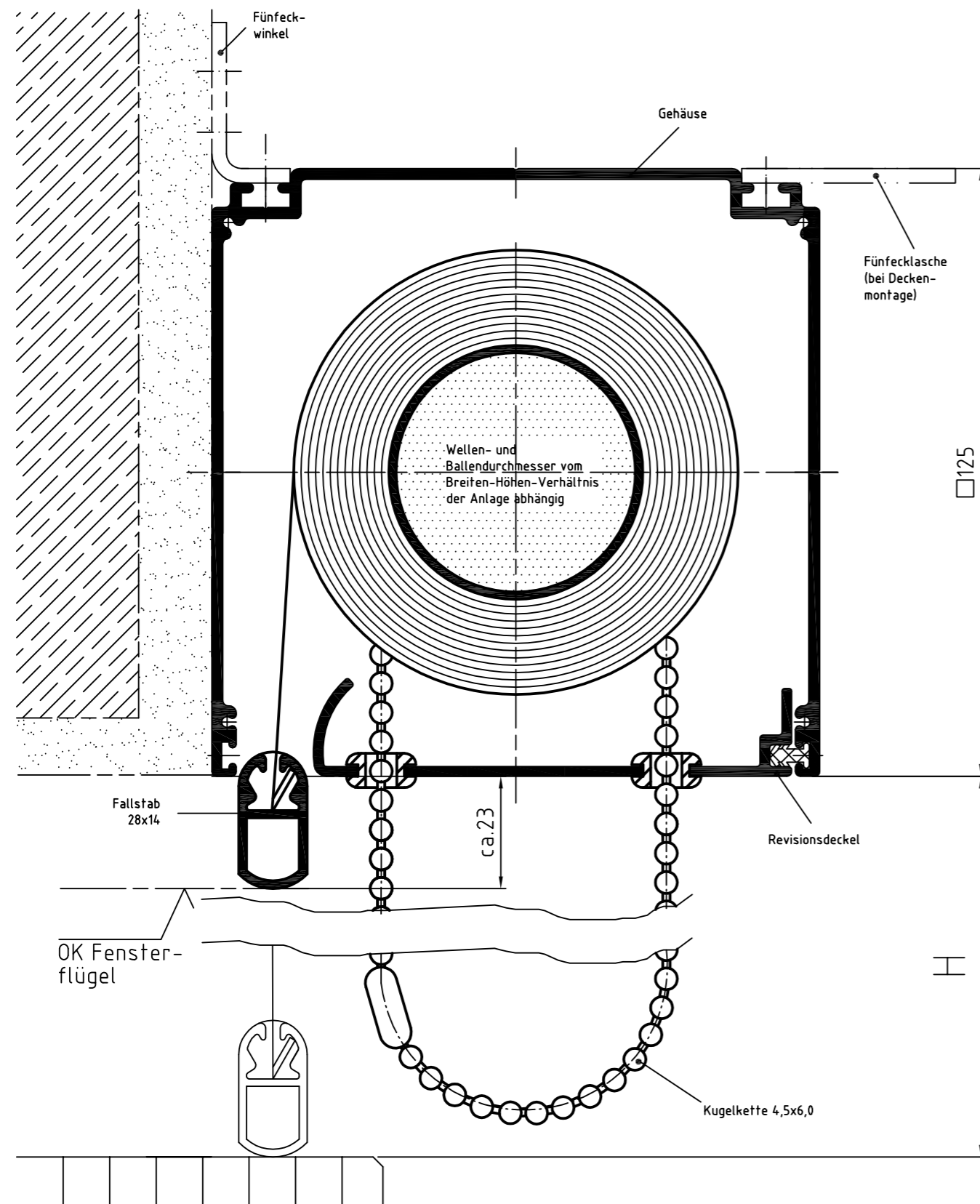
Zeichnung KQ 125 – Querschnitt Systemskizze | ohne Maßstab | sämtliche Angaben in mm
