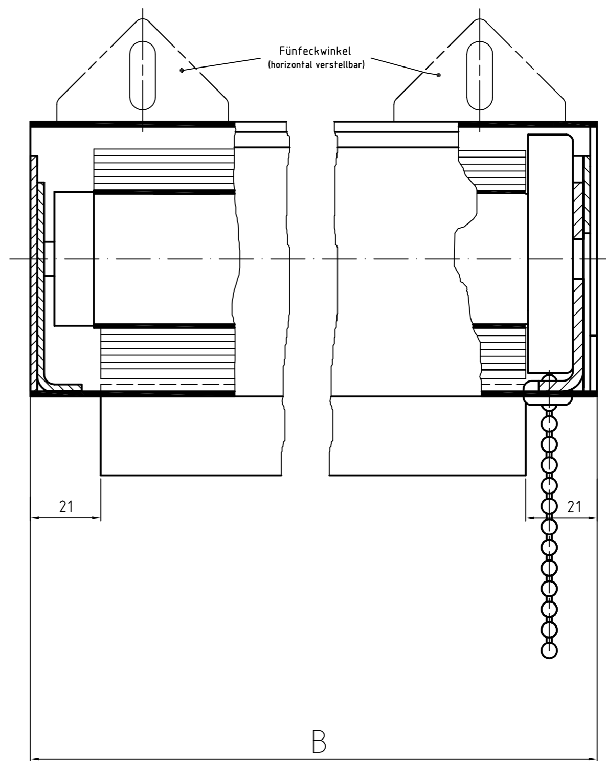
Zeichnung KQ 80 – Längsschnitt Systemskizze | ohne Maßstab | sämtliche Angaben in mm
