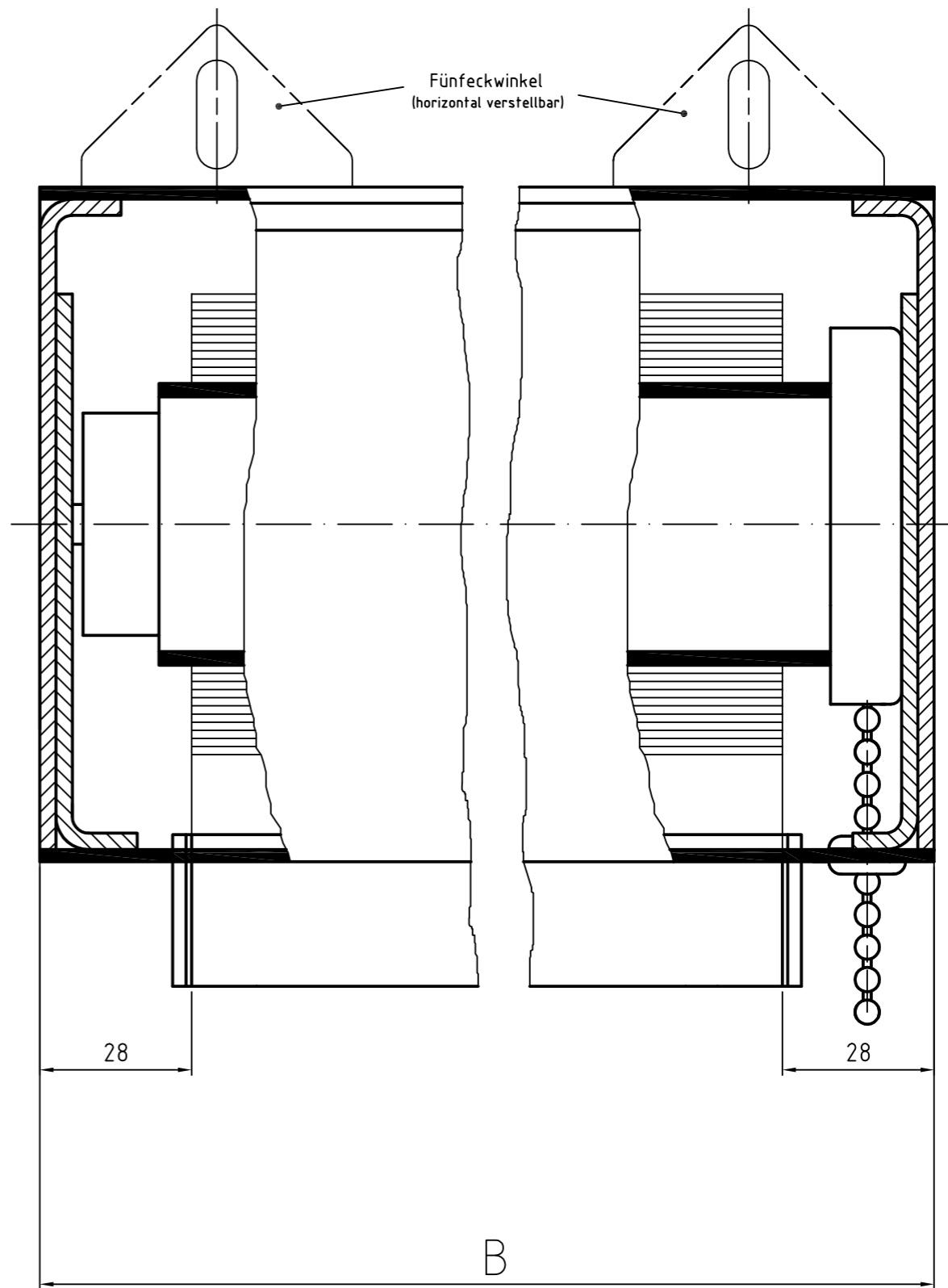
Zeichnung KQ 125 – Längsschnitt Systemskizze | ohne Maßstab | sämtliche Angaben in mm
