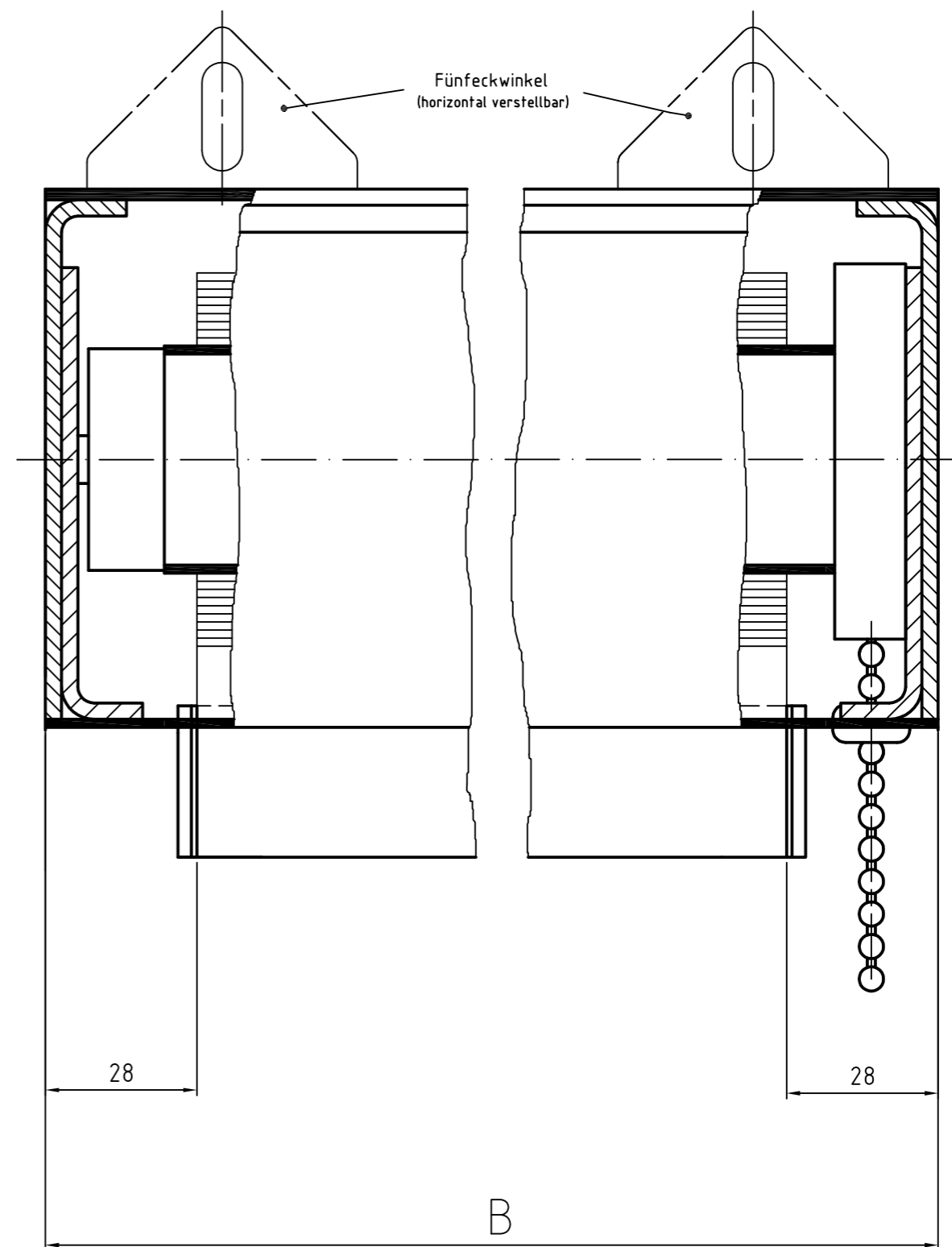
Zeichnung KQ 100 – Längsschnitt Systemskizze | ohne Maßstab | sämtliche Angaben in mm
