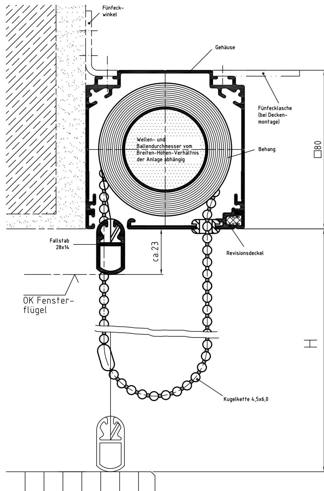
Zeichnung KQ 80 – Querschnitt Systemskizze | ohne Maßstab | sämtliche Angaben in mm
