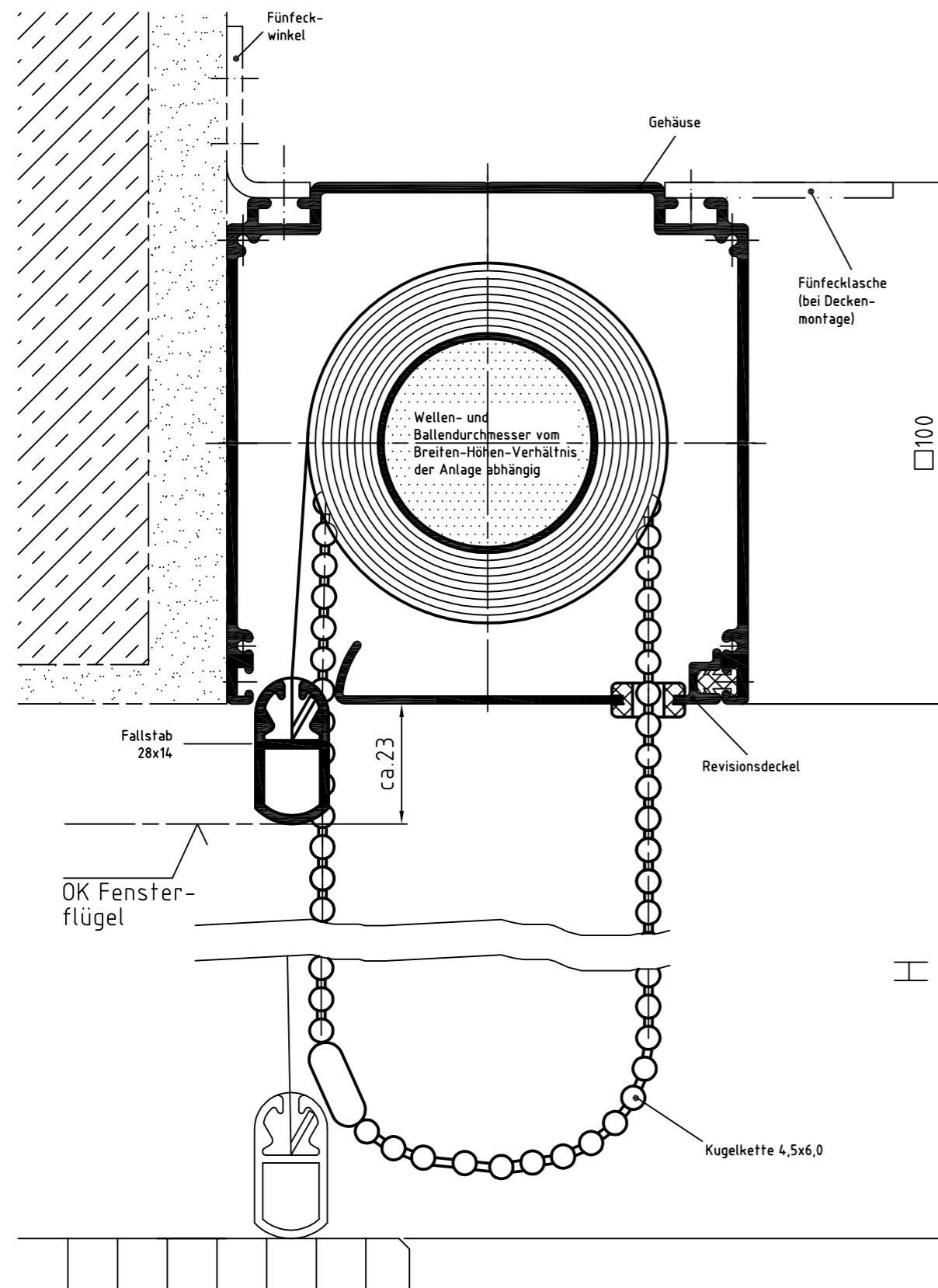
Zeichnung KQ 100 – Querschnitt Systemskizze | ohne Maßstab | sämtliche Angaben in mm
