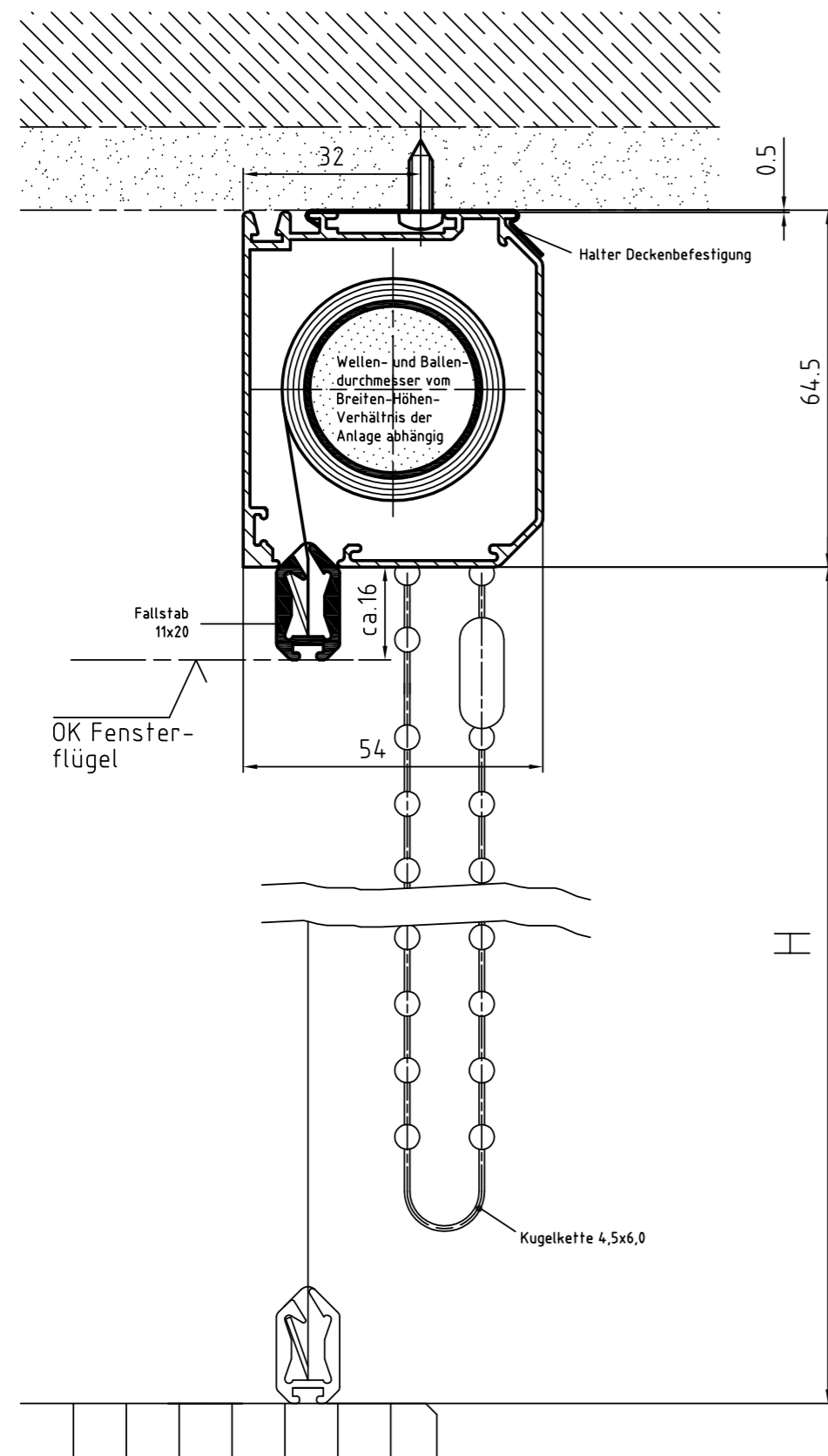
Zeichnung KQ 60 – Querschnitt Systemskizze | ohne Maßstab | sämtliche Angaben in mm
