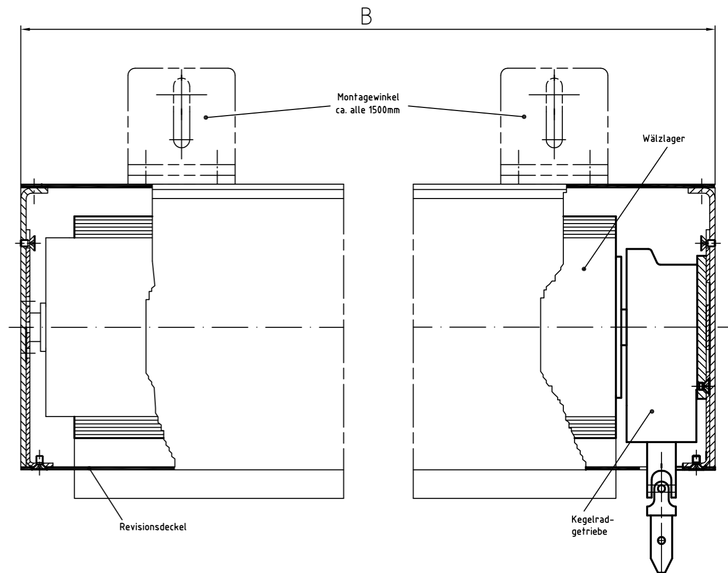
Zeichnung GQ 160 – Längsschnitt Systemskizze | ohne Maßstab | sämtliche Angaben in mm
