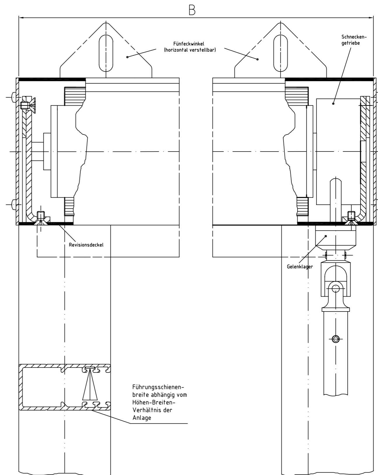
Zeichnung GQ 80 – Längsschnitt Systemskizze | ohne Maßstab | sämtliche Angaben in mm
