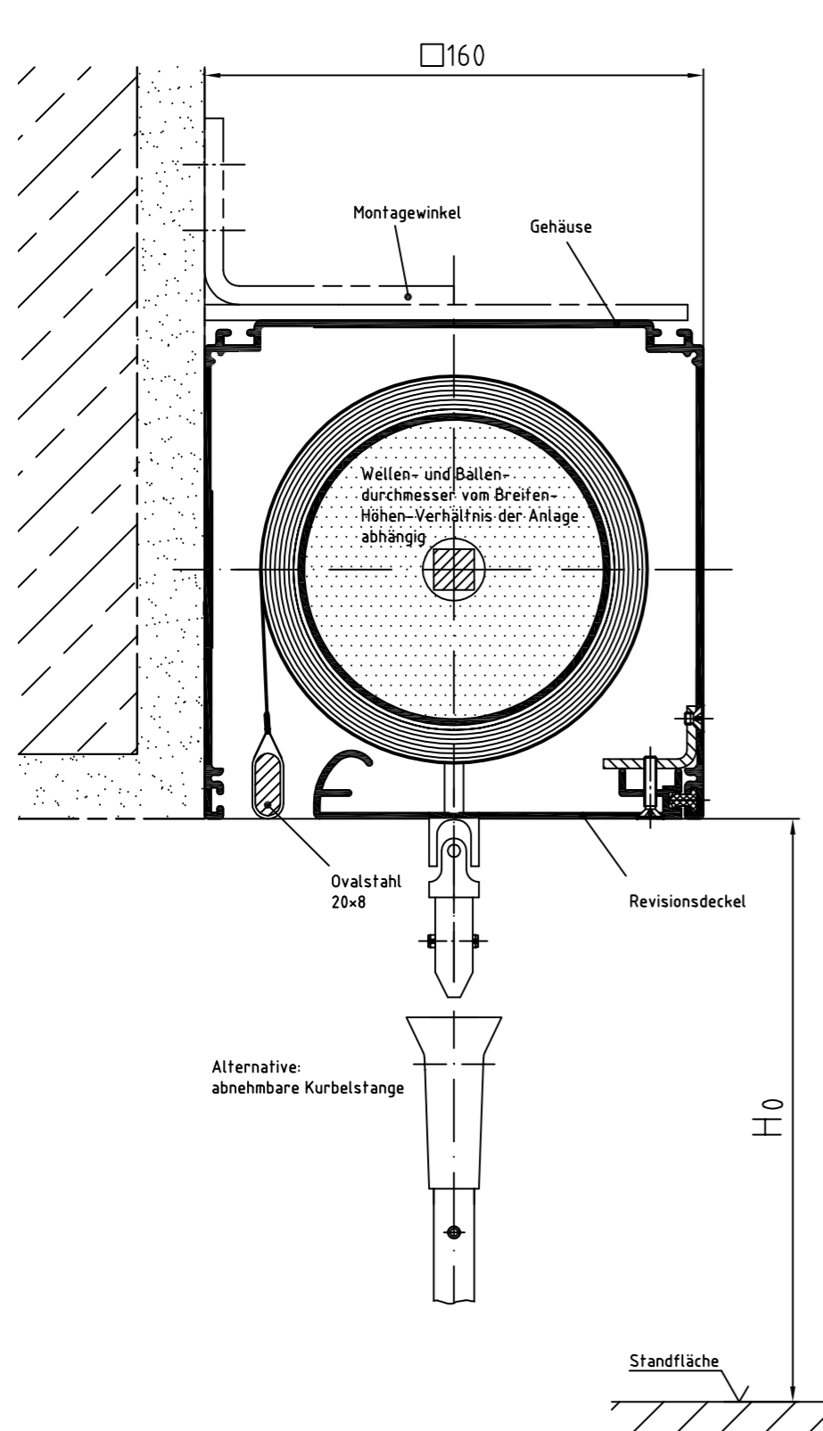
Zeichnung GQ 160 – Querschnitt Systemskizze | ohne Maßstab | sämtliche Angaben in mm
