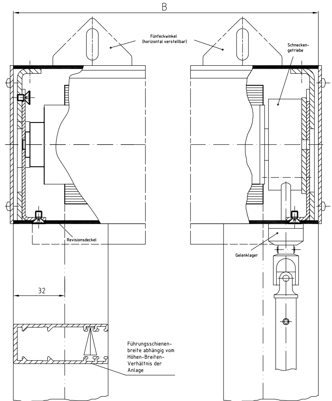
Zeichnung GQ 100 – Längsschnitt Systemskizze | ohne Maßstab | sämtliche Angaben in mm
