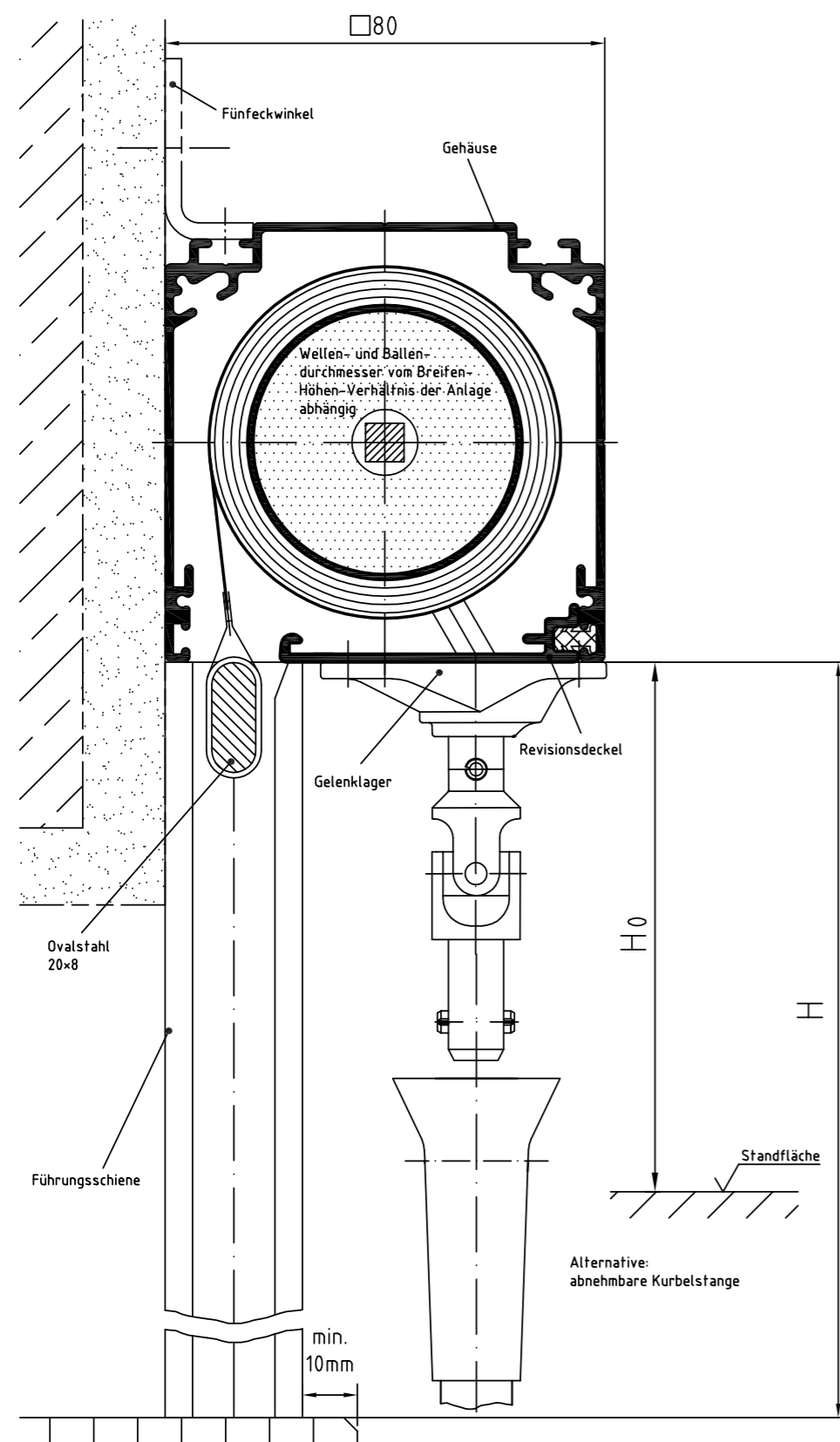
Zeichnung GQ 80 – Querschnitt Systemskizze | ohne Maßstab | sämtliche Angaben in mm
