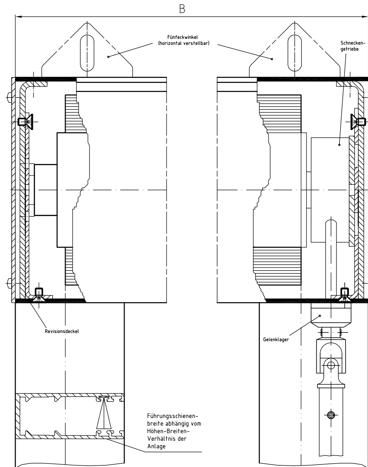
Zeichnung GQ 125 – Längsschnitt Systemskizze | ohne Maßstab | sämtliche Angaben in mm
