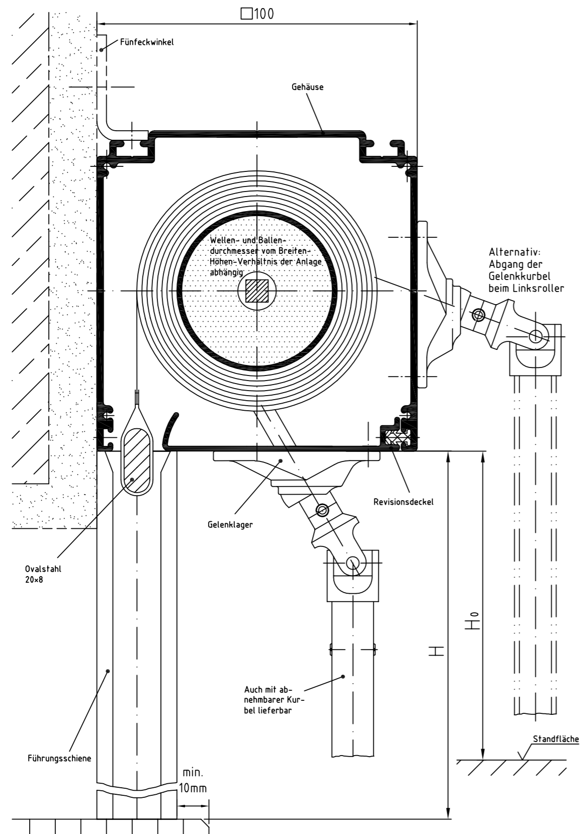
Zeichnung GQ 100 – Querschnitt Systemskizze | ohne Maßstab | sämtliche Angaben in mm
