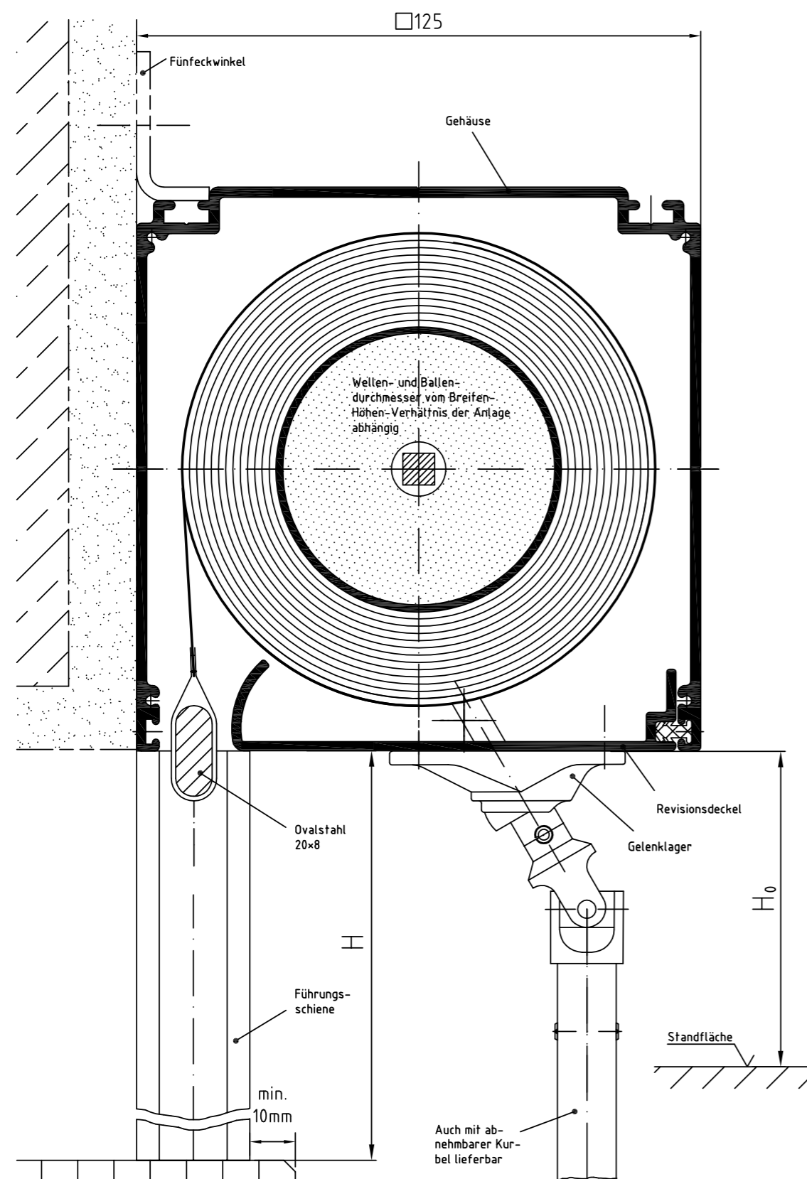
Zeichnung GQ 125 – Querschnitt Systemskizze | ohne Maßstab | sämtliche Angaben in mm
