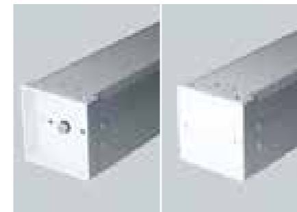
Montagefreundliche Aufhängung dank verformungsstabiler Alu-Gusskopfstücke oder Stahl-Lagerwinkel mit verdeckter Befestigung.
