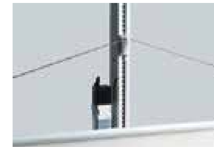
Gegenzuganlage mit Tuchspannung durch Federwellenmechanismus und Linearantrieb (Helsinki, Oslo).
