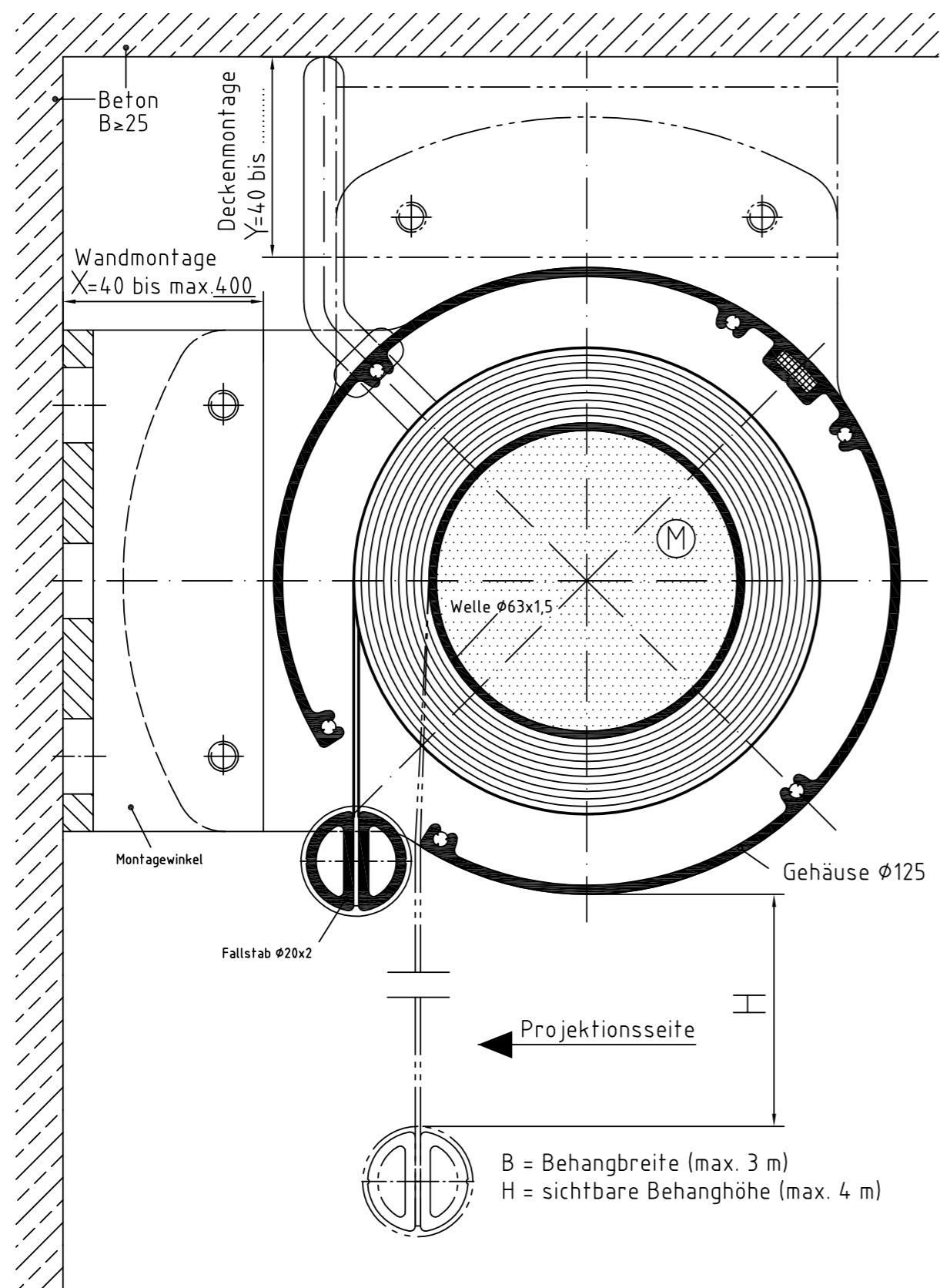
Zeichnung BW-MR 125 – Querschnitt Systemskizze | ohne Maßstab | sämtliche Angaben in mm
